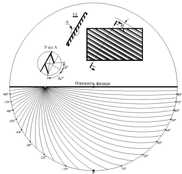
Рисунок И.4 – Теневой угломер для расчета СЗУ общего положения восточной ориентации при угле наклона направляющей ламелей 30^\circ
