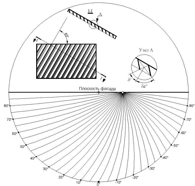
Рисунок И.3 – Теневой угломер для расчета СЗУ общего положения западной ориентации при угле наклона направляющей ламелей 60^\circ
