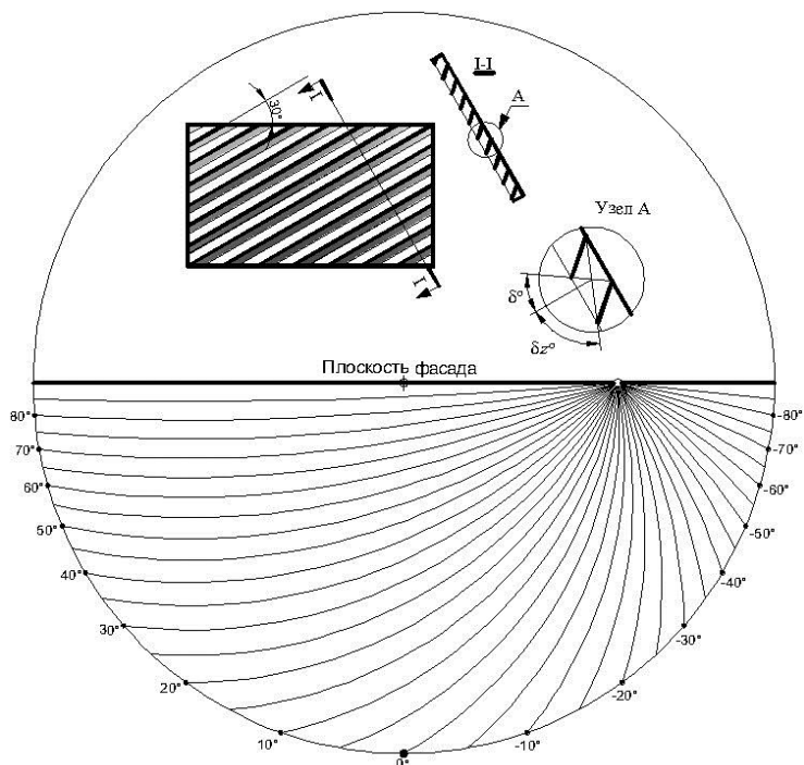
Рисунок И.2 – Теневой угломер для расчета СЗУ общего положения западной ориентации при угле наклона направляющей ламелей 30^{\circ}
