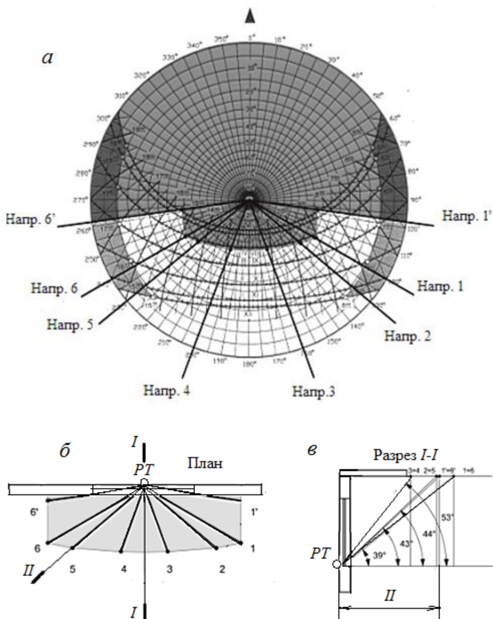
a – солнечная карта для 52° с.ш.; б – план козырька; в – разрез козырька; Напр. – азимутальное направление
