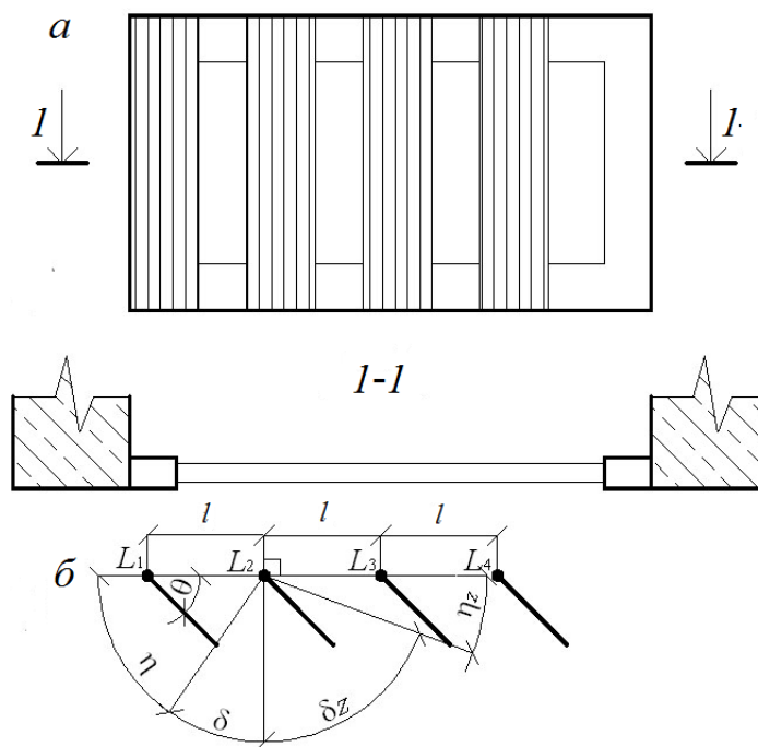
Рисунок Ж.6 – Параметры проектируемого солнцезащитного устройства с вертикальными ламелями
